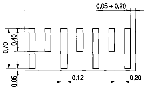
2.1. Wymiary odcinków linii i odstępów, stanowiących znak P-25 („próg zwalniający”)
