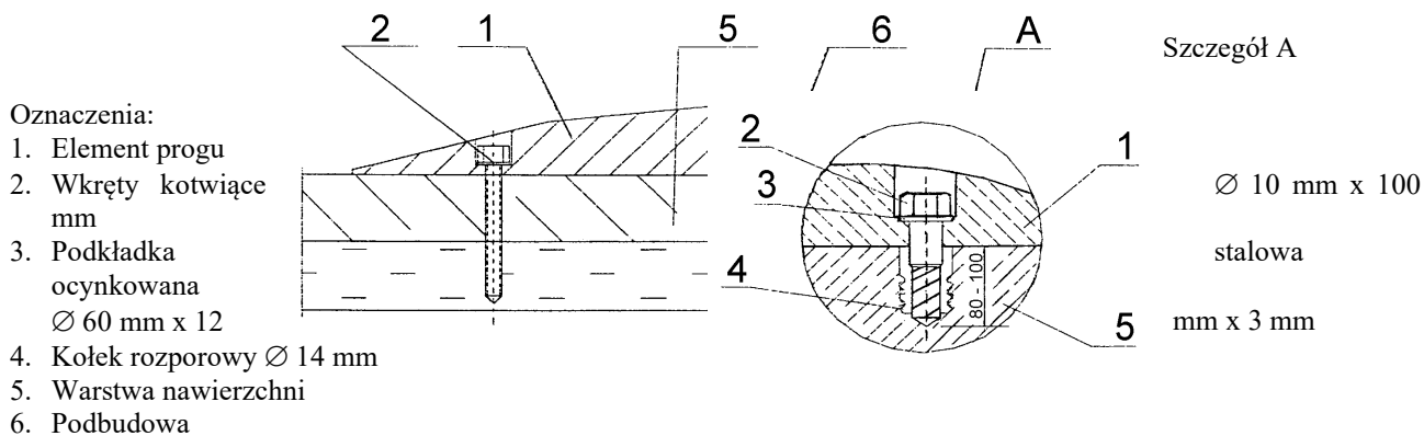
Rys. 4. Przykład umocowania progu do nawierzchni jezdni
