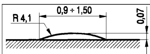
Rys. 4. Przekrój podłużny liniowego progów zwalniającego listwowego o ograniczonej prędkości przejazdu 18 ÷ 20 km/h (U-16d)
