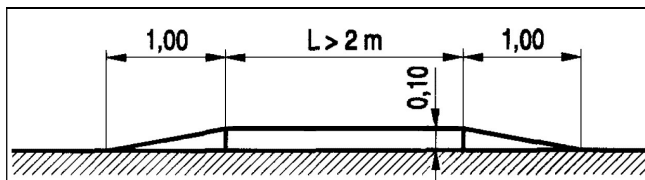
Rys. 4. Przekrój podłużny liniowego progów zwalniającego listwowego o ograniczonej prędkości przejazdu 18 ÷ 20 km/h (U-16d)
