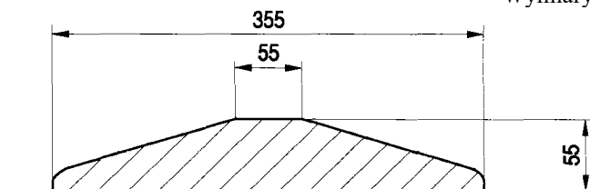
KSZTAŁT I WYMIARY W PRZEKROJU POPRZECZNYM PRZYKŁADOWYCH PROGÓW PODRZUTOWYCH (wg [23]) Wymiary w mm
