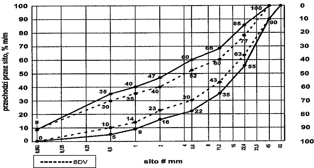
Rys. 2. Krzywe graniczne uziarnienia mieszanki kruszywa niezwiązanego 0/45 mm zasadniczej
