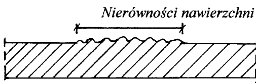
Rys. 2. Schemat przekrojów poprzecznych nawierzchni, w której wyrównano asfaltem lanym lokalne nierówności
